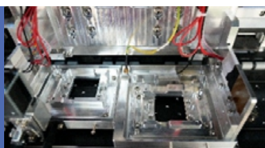
Riscaldamento base carrello
